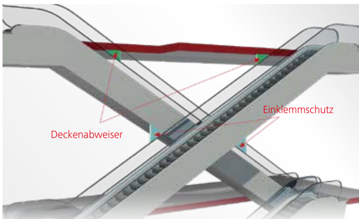
Einklemmschutz
