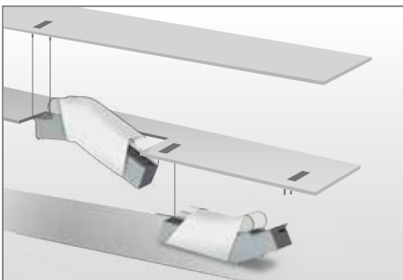
Montage in mehreren Teilen
