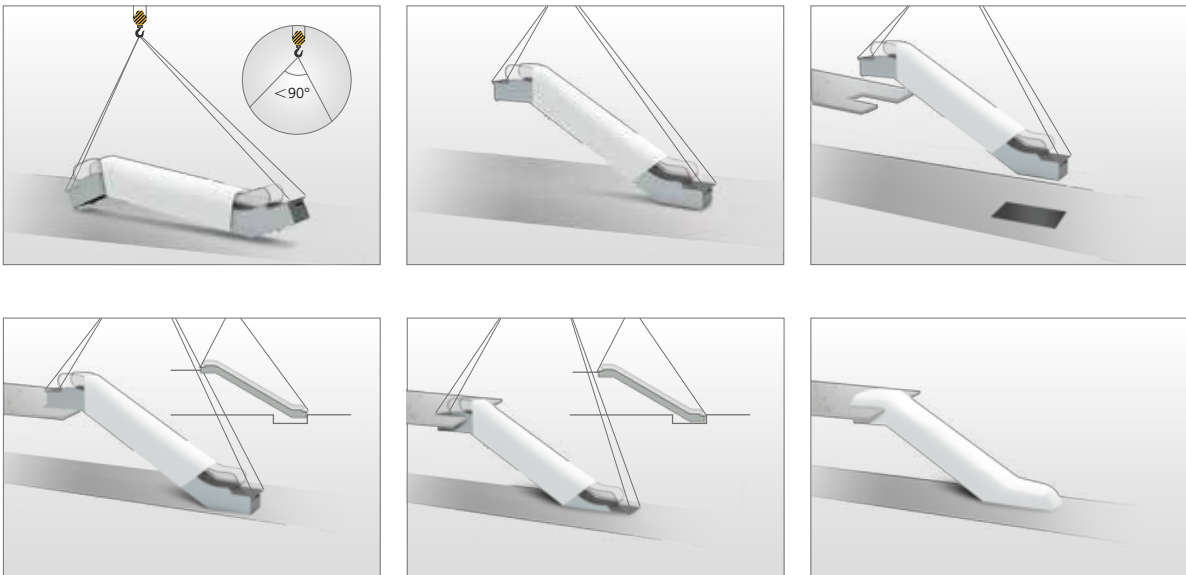
Montage der Anlage in einem Stück mittels Kran
