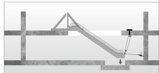
Montage der Anlage in einem Stück mittels Gerüsten
