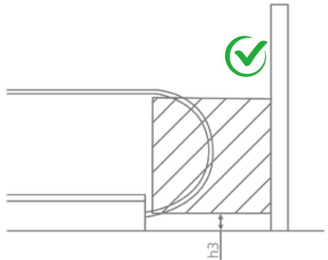
Abb. 6d: Höhe der Unterkante der zusätzlichen Barriere > tatsächlicher Wert h_3
