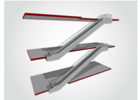
Unterbrochene Anordnung (Verkehr in eine Richtung)
