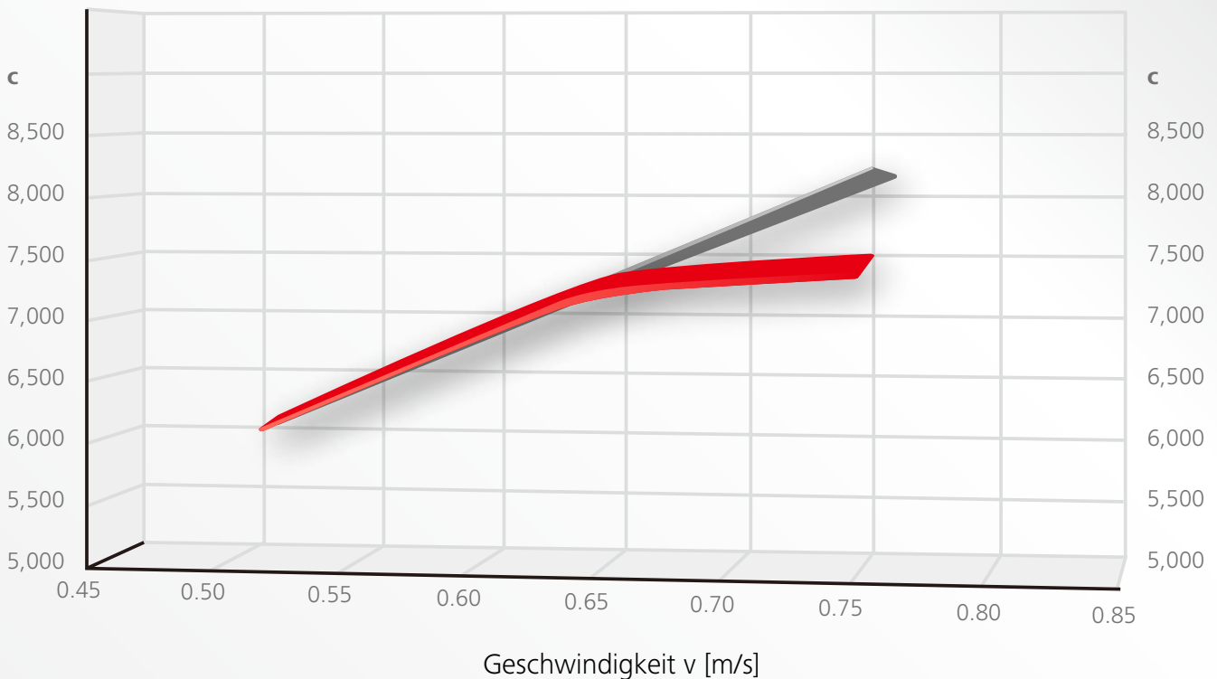
Förderleistung c (Personen/h) in Abhängigkeit von der Fahrgeschwindigkeit c = theoretische Förderleistung (Personen/h) bei Nennbreite 1.000 mm
